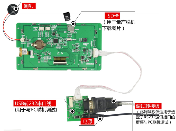
图 1-5 调试工具图
