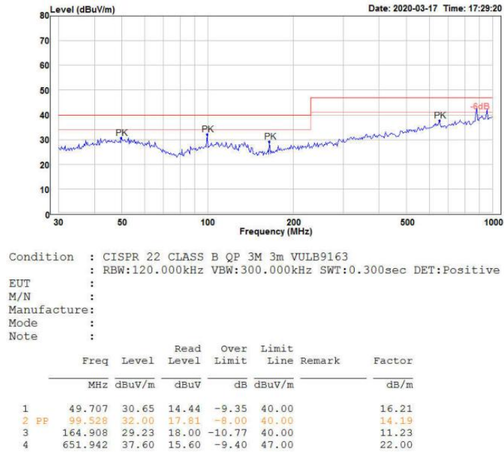
图 4-5 RE 测试水平方向
