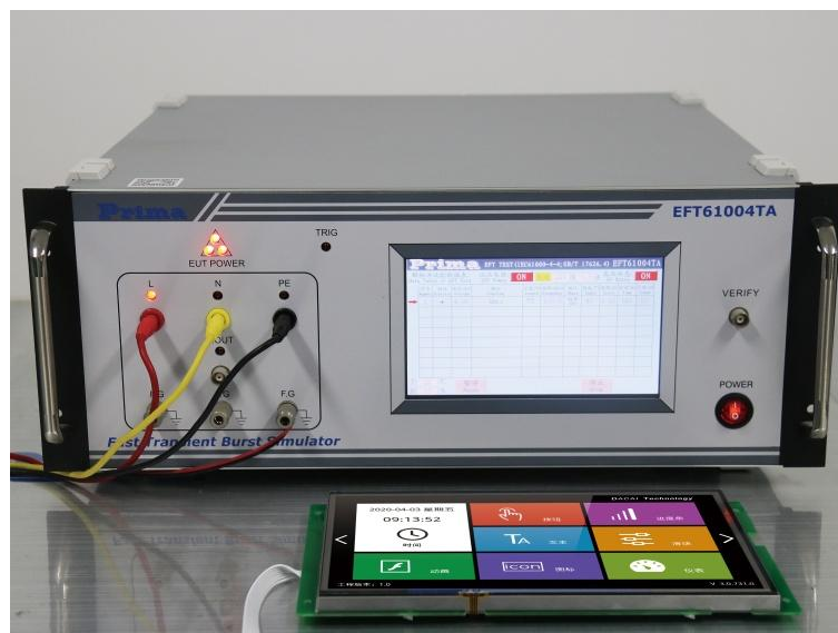
图 4-3 EFT 测试图
